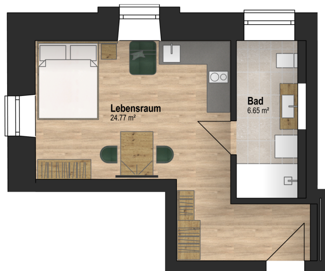
Wohnung 6 31.42 m², Obergeschoss, Ausrichtung Nord-West
