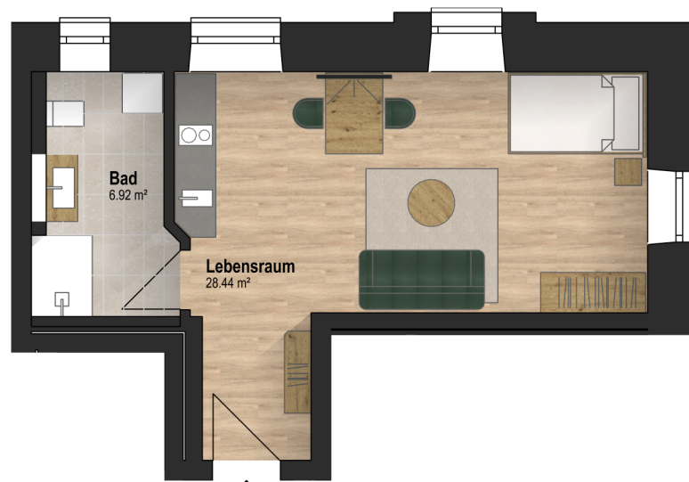
Wohnung 7 35.36 m 2 , Obergeschoss, Ausrichtung Nord-Ost
